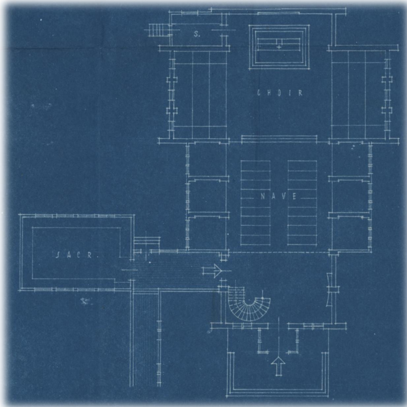
P61:4.11-02/01 Extrait du dessin d'architecture.
